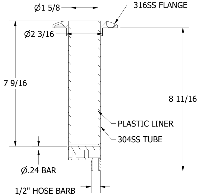
SECTION A-A
