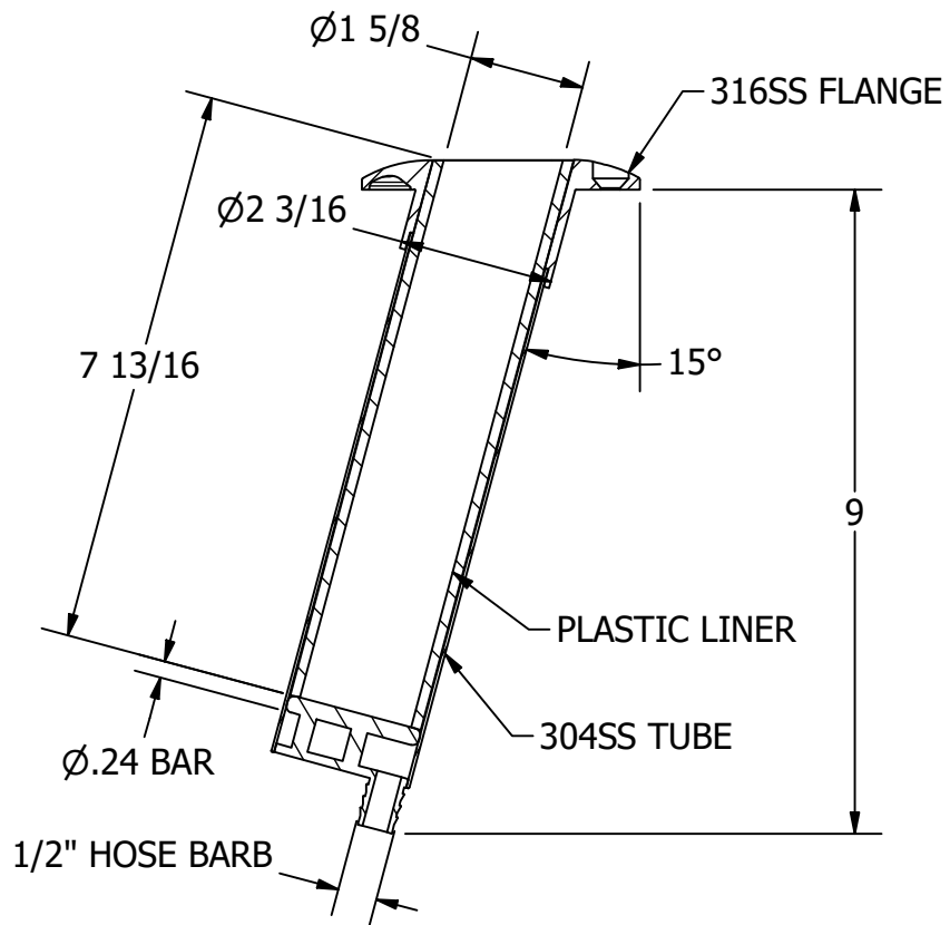
SECTION A-A
