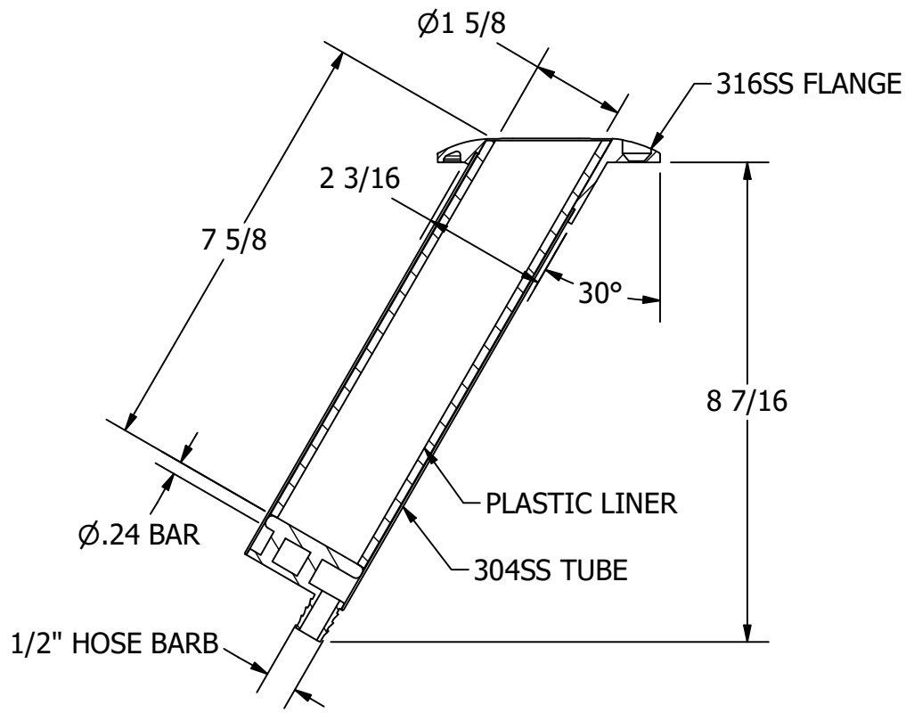
SECTION A-A
